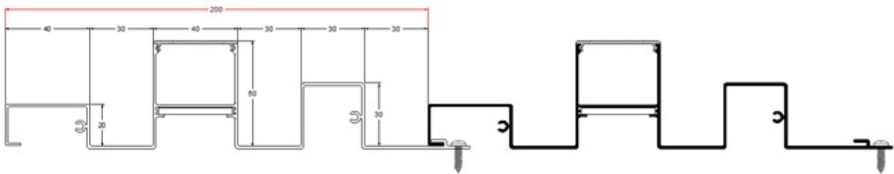
WD-5000 dikte 1,2 mm
